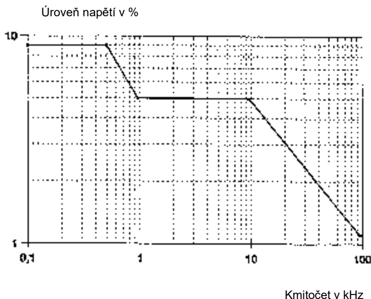
Obrázek 1 – Úrovně napětí na kmitočtech signálů v procentech U_c ve veřejných distribučních sítích vn
