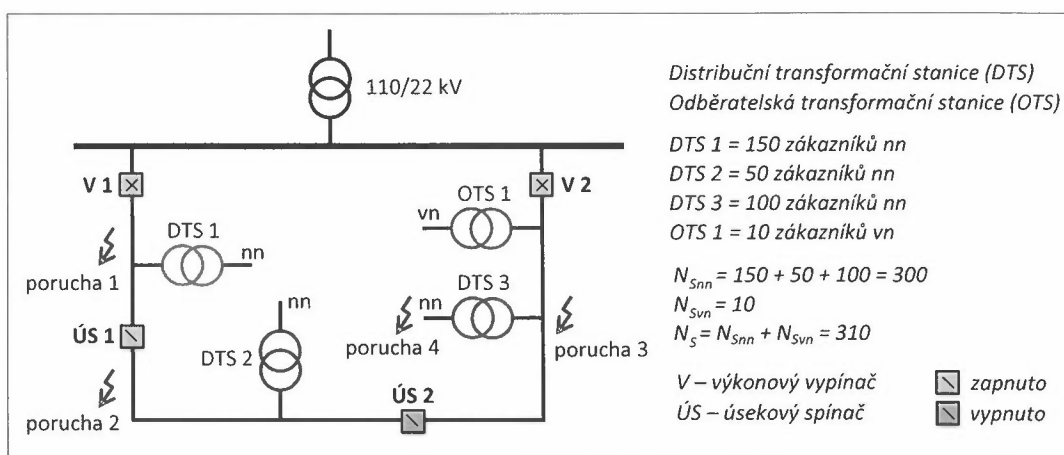
Obr. 1: Schéma distribuční soustavy
