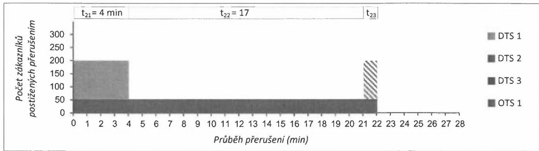
Obr. 8: Grafický průběh přerušení při poruše 2
