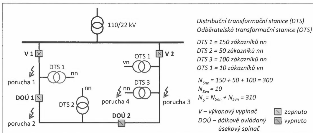
Obr. 6: Schéma distribuční soustavy
