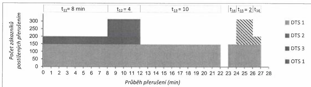
Obr. 2: Grafický průběh přerušení při poruše 1
